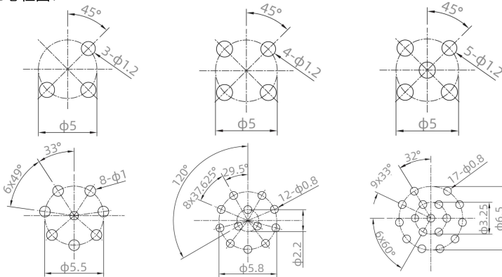
PCB芯位图:
